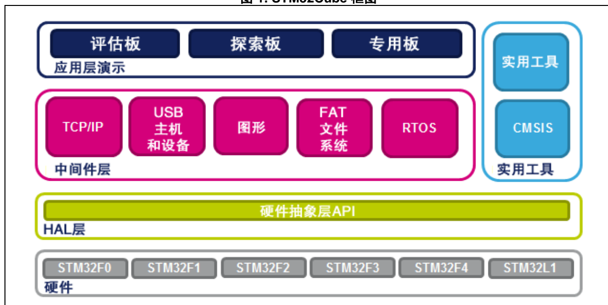
图 1. STM32Cube 框图
