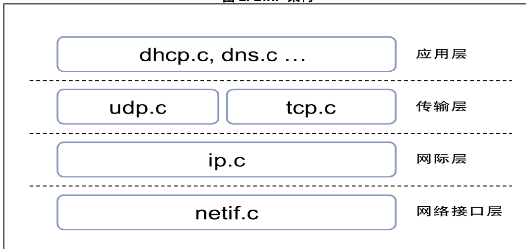
图 2. LwIP 架构
