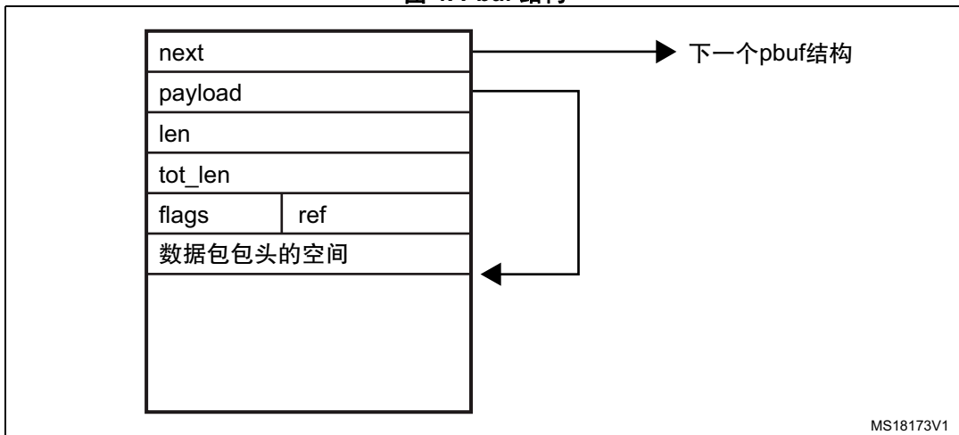
图 4. Pbuf 结构
