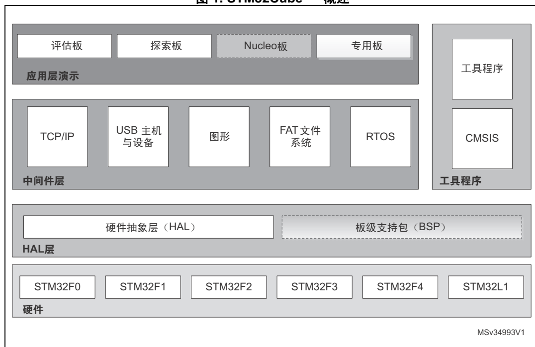
图 1. STM32Cube™ 概述
