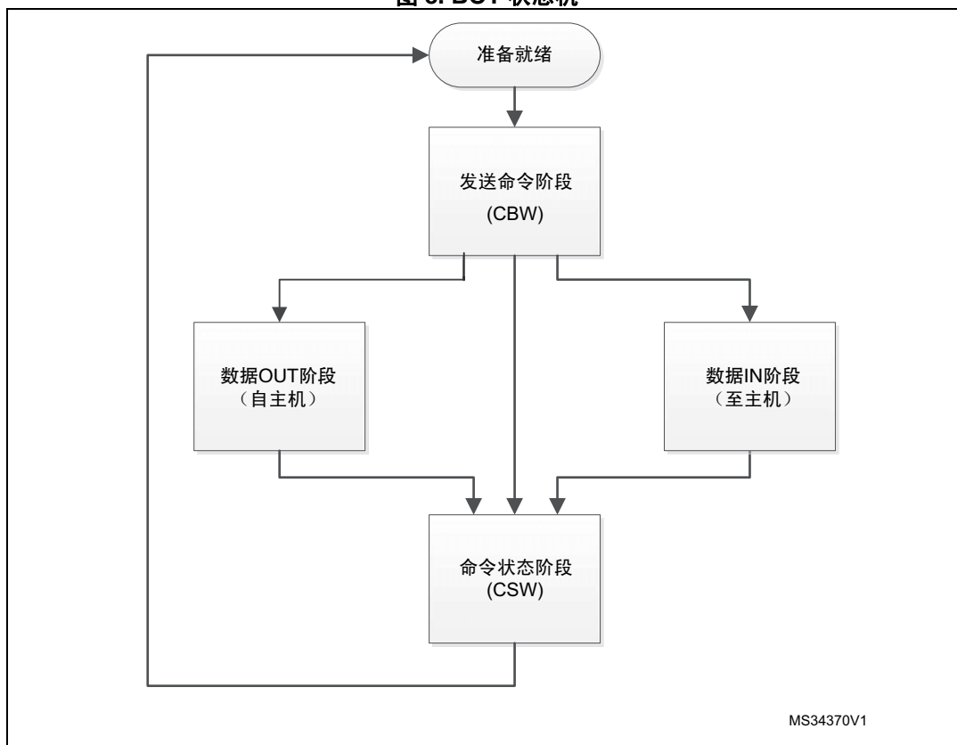
图 8. BOT 状态机
