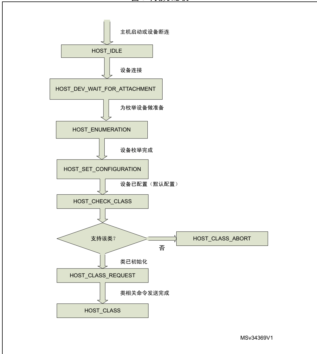
图 6. 内核状态机
